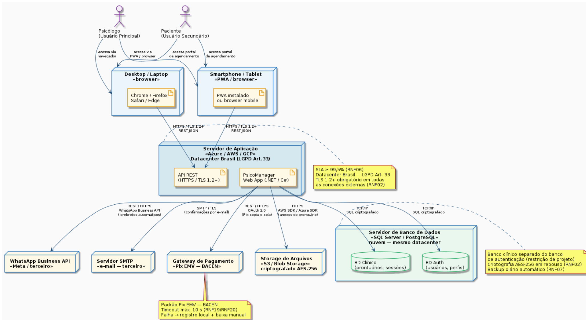
Figura: C1 — Diagrama de Implantação · Arquivo: C1_Implantacao.puml
